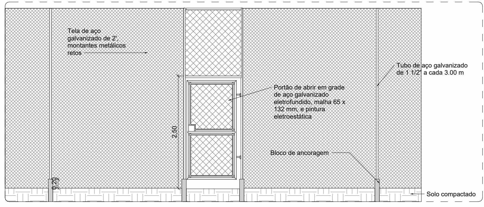
5 DETALHAMENTO DE ALAMBRADO E PORTÃO 1 FOLHA 1 : 50
