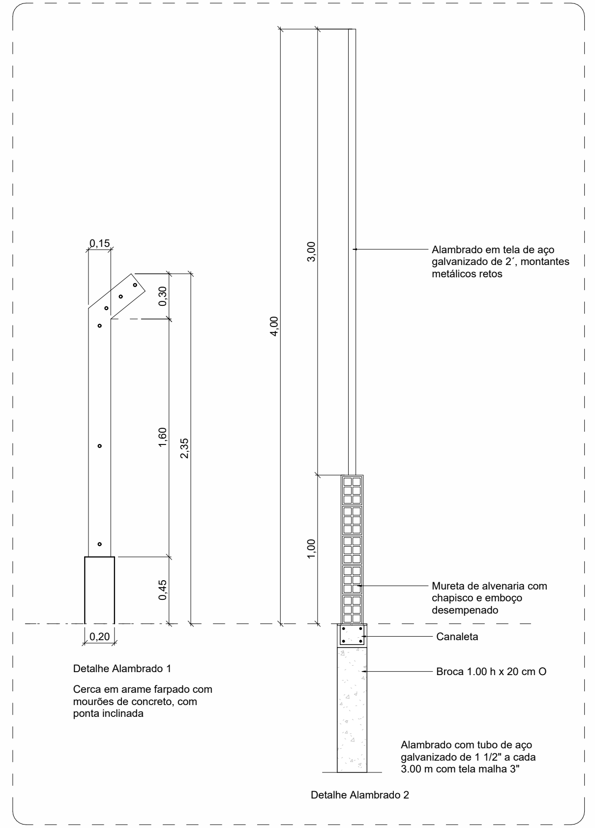
8 DETALHAMENTO - ALAMBRADOS 1 : 25
