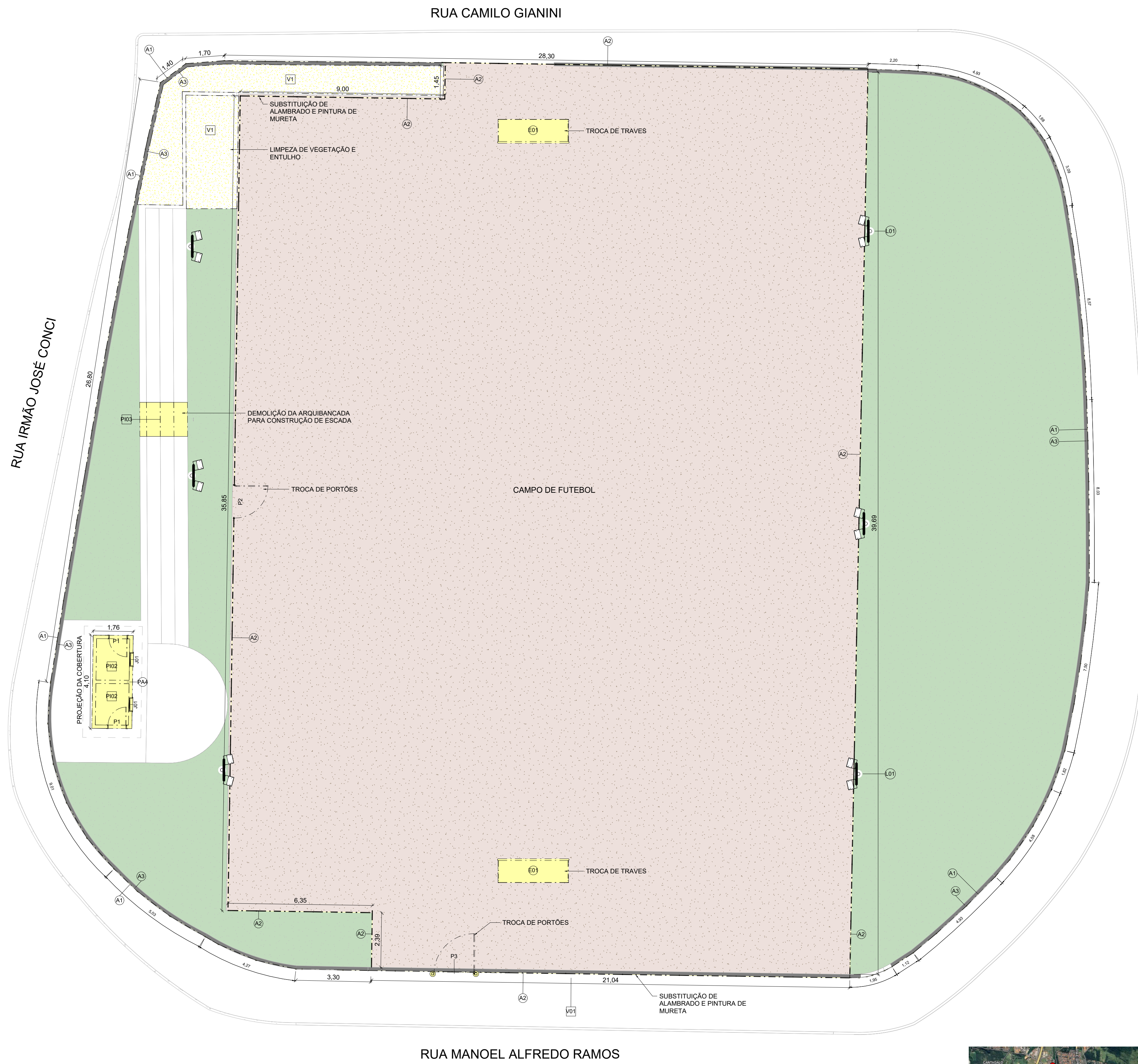
3 PLANTA DE COBERTURA - DEMOLIÇÃO 1 : 100
