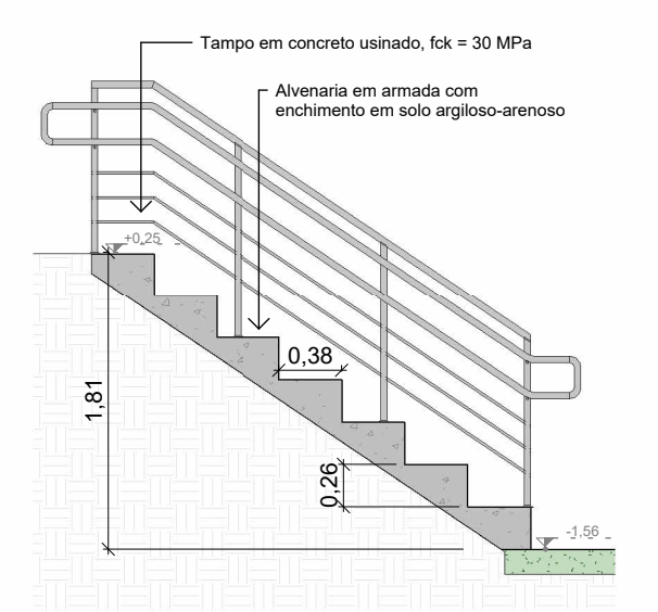
3 DETALHAMENTO ESCADA 1 : 50
