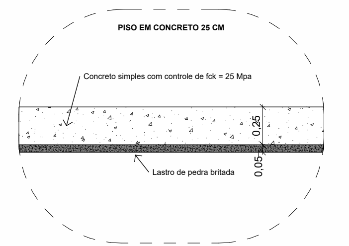
4 DET. PISOS 1 : 25
