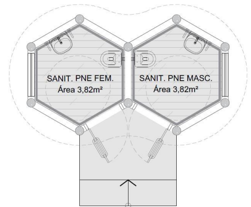
PLANTA BAIXA - SANITÁRIOS
