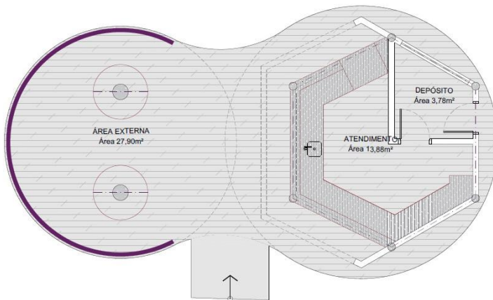
PLANTA BAIXA - QUIOSQUE 02
